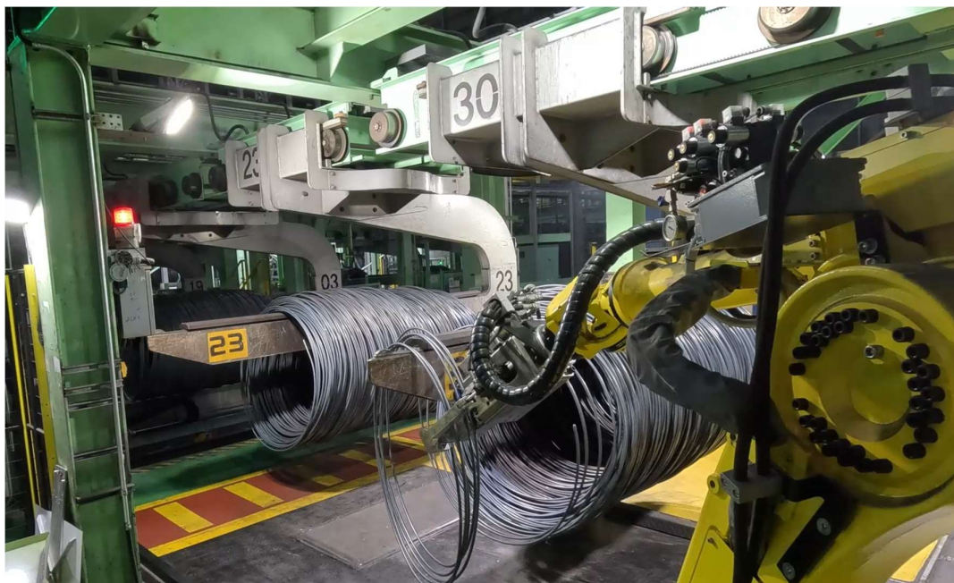
Автономный робот TrimRob для обрезки бунтов и отбора проб от Primetals Technologies
